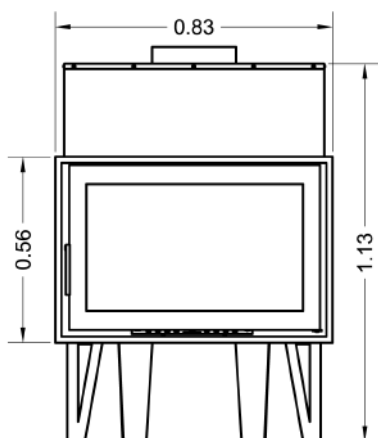
Μπροστινή Όψη
