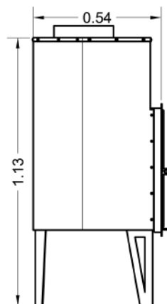
Πλάγια Όψη
