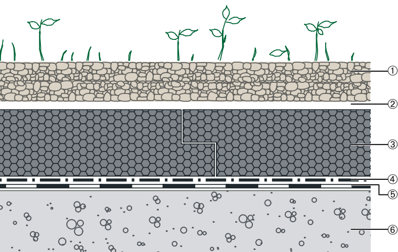
Φυτεμένο δώμα εκτακτικής φύτευσης
