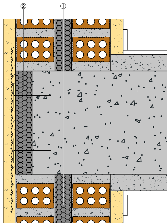
Θερμομόνωση σε διπλό τοίχο και φέροντα οργανισμό
